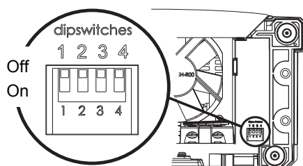
Afbeelding 7: DIP-switches
