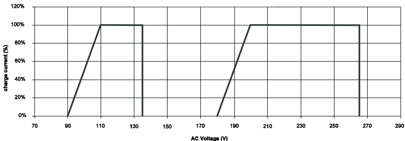
Afbeelding 14: Laadstroom (charge current) versus ingangsspanning (AC voltage)
